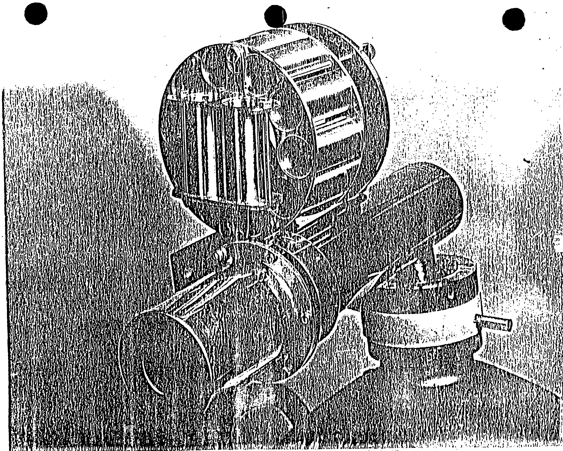
Fig. III-A. Holder for Ge(Li) detector system.
